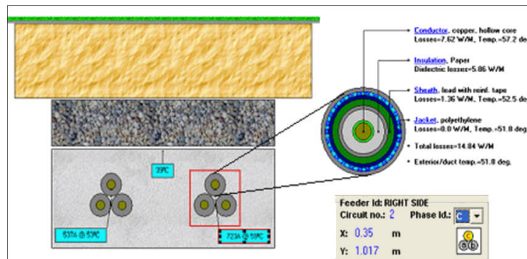
Modèle CYMCAP et résultats pour une installation multicouche
